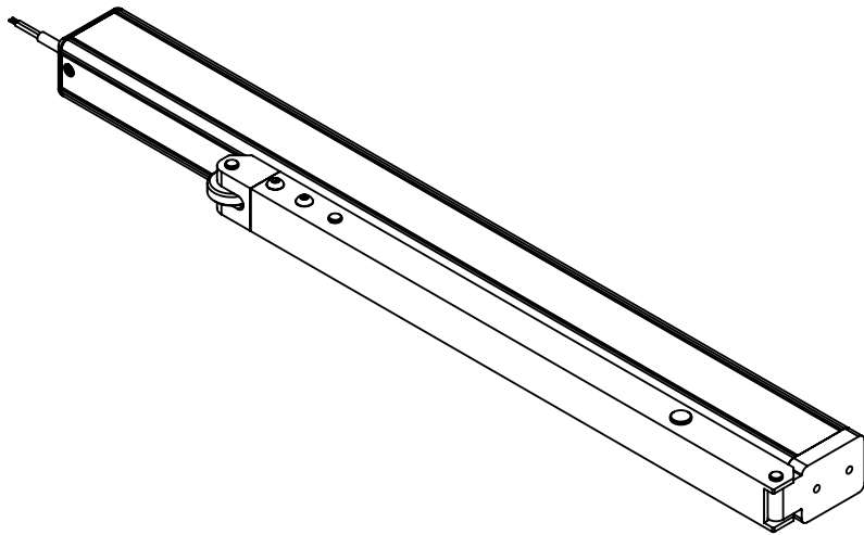
AFSl 04009 RS Isometric SCALE 1 : 5
