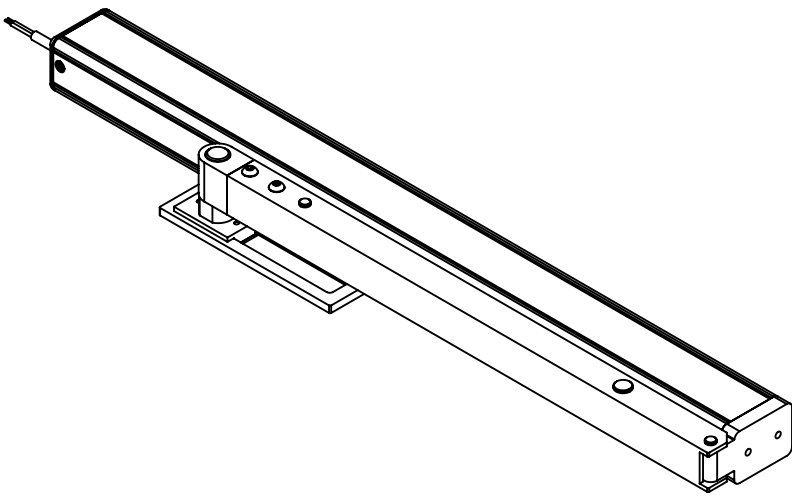
AFSl 04009 FS Isometric SCALE 1 : 5
